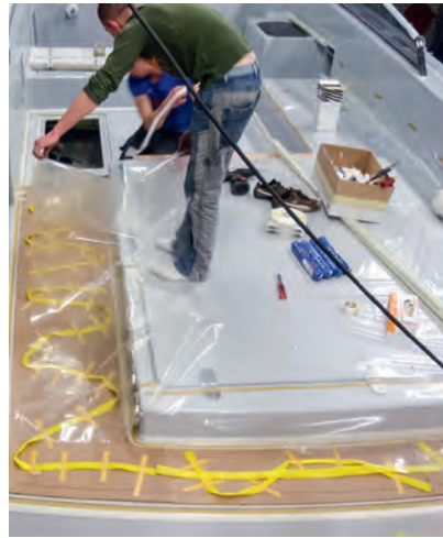
Fig. 15 Vacuum press
